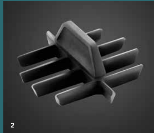
1 La piletta dello scarico della doccia è facilmente removibile. 2 Il pratico inserto a pettine può essere rimosso facilmente e risciacquato secondo le necessità, garantendo così anche il perfetto funzionamento dello scarico.
